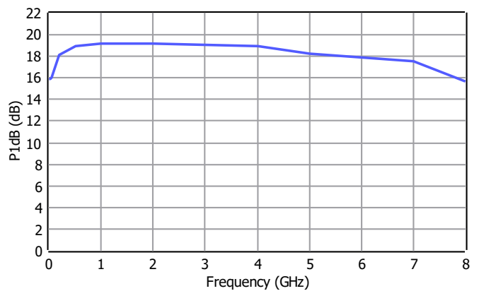
P1dB
